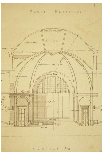
图15 大礼堂剖面设计图，图中小字可辨认“Guastivino Dome & Ribs”，拼写有误，第1个“i”应作“a”。
