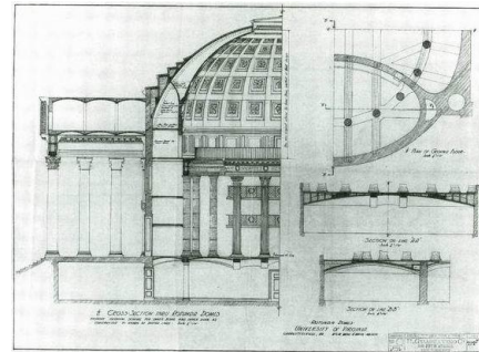
图9 重建的圆厅图书馆剖面设计图, 1903
